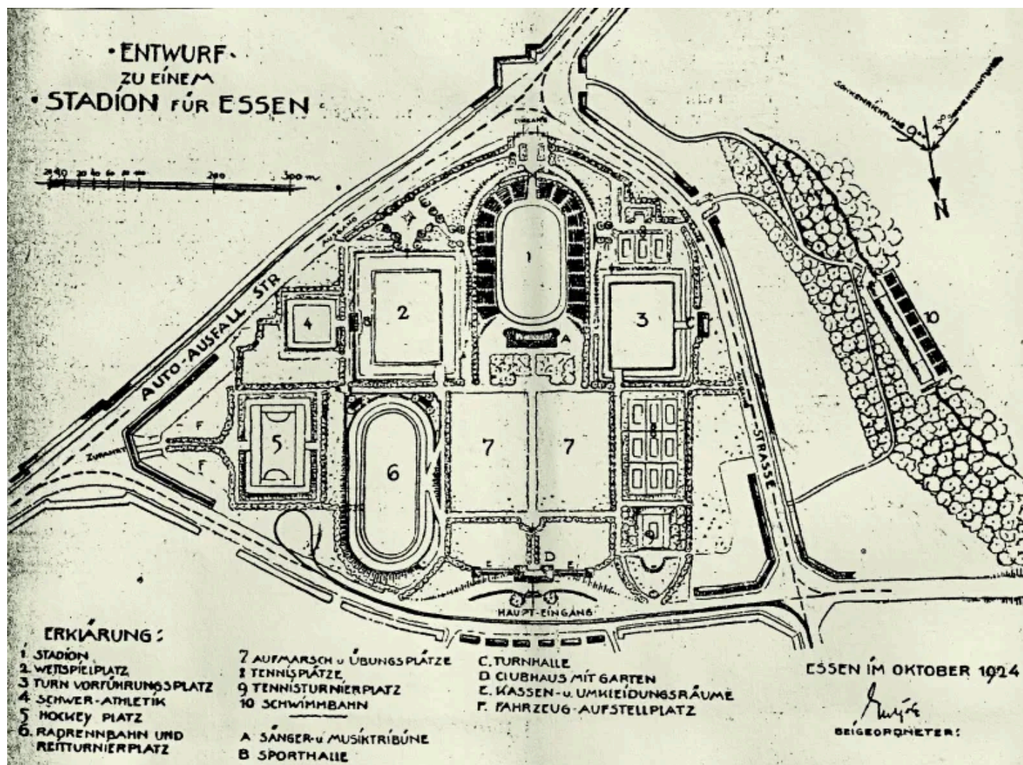
Entwurf zu einem Stadion für Essen aus dem Jahre 1924.
